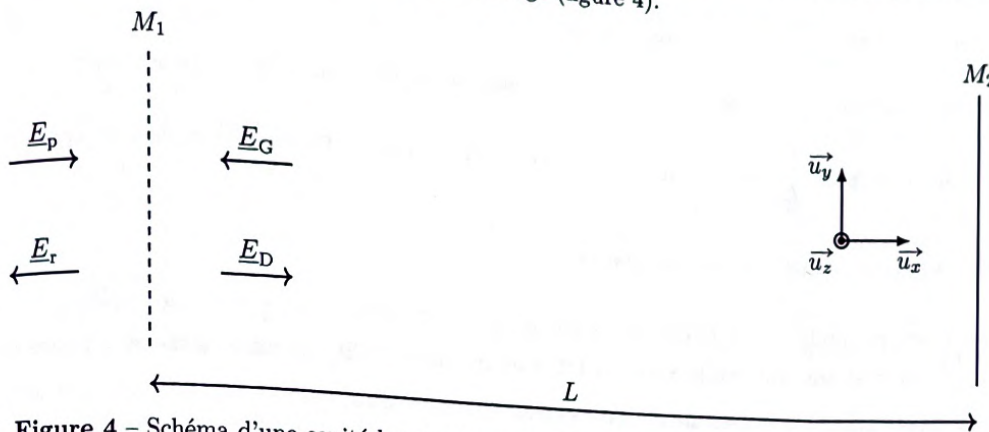
Figure 4 – Schéma d'une cavité laser avec pertes. Les flèches sous les amplitudes complexes des champs électriques indiquent la direction et le sens de propagation des ondes associées.
