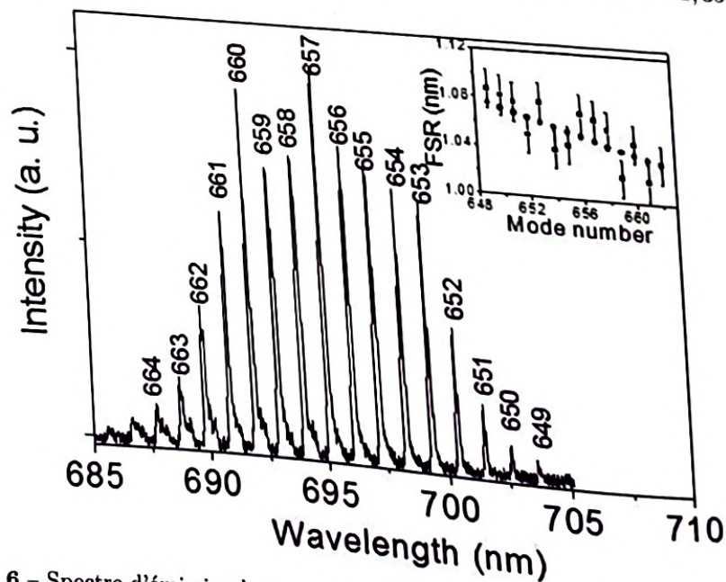
Figure 6 – Spectre d'émission laser expérimental de Lahoz et al. [2] en longueur d'onde. L'intensité est en unité arbitraire. Les différents modes du rayonnement sont précisés par les numéros de mode portés au-dessus des pics correspondants. L'insert représente l'Intervalle Spectral Libre en longueur d'onde ( FSR_\lambda ) en fonction du numéro de mode.
