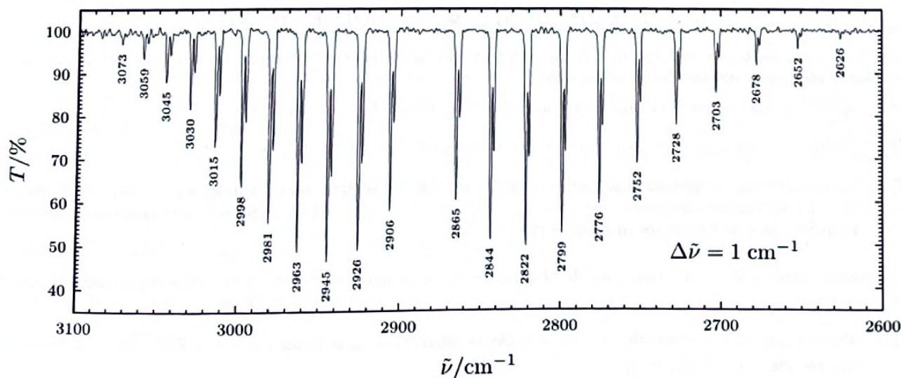
Figure 3 – Spectre de transmittance de HCl produit par FTIR [1]. Les nombres d'onde de certaines transitions sont indiqués (le nombre d'onde, noté ici \tilde{\nu} , est l'inverse de la longueur d'onde). Leurs incertitudes-types associées sont de 1 \text{ cm}^{-1} . Aucune raie d'absorption n'est observée en dehors de l'intervalle de mesure présenté.
