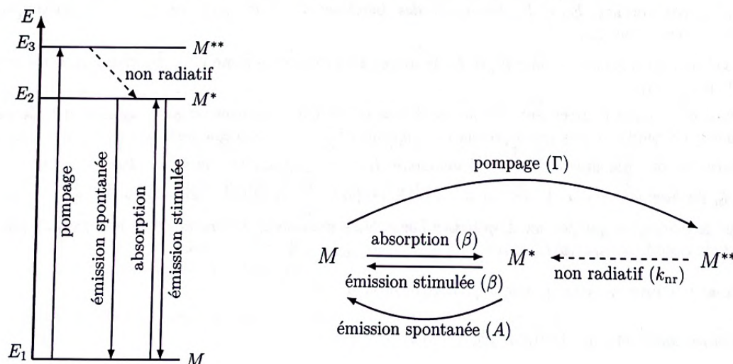
Figure 5 – Gauche : Diagramme des états d'énergie de l'espèce M présente dans le milieu amplificateur et transitions possibles.
