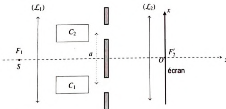
Figure 10 - Montage interférentiel
