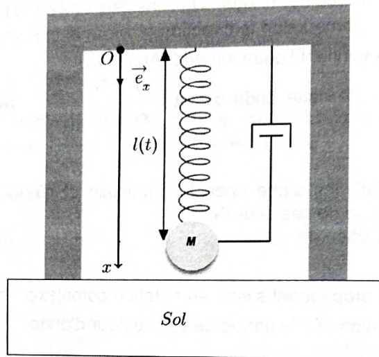
Figure 3 - Sismomètre
