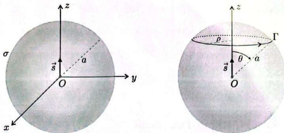
FIGURE 1 – Le dipôle \vec{s} , la coquille chargée et le cercle \Gamma .
