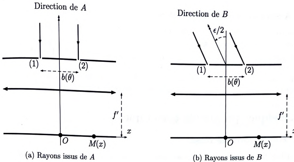
FIGURE 3 – Représentation schématique d'un télescope double
