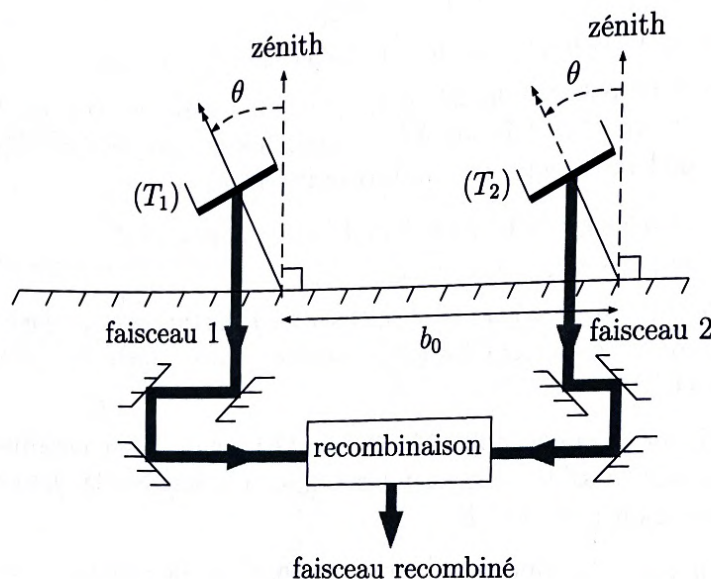
FIGURE 2 – Représentation d'un télescope double
