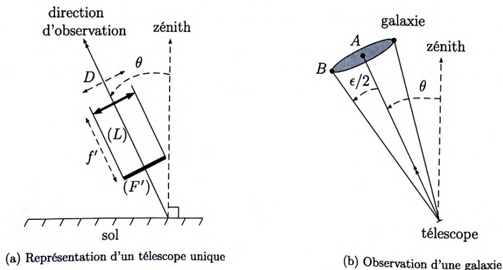
FIGURE 1 – Modélisation du dispositif
