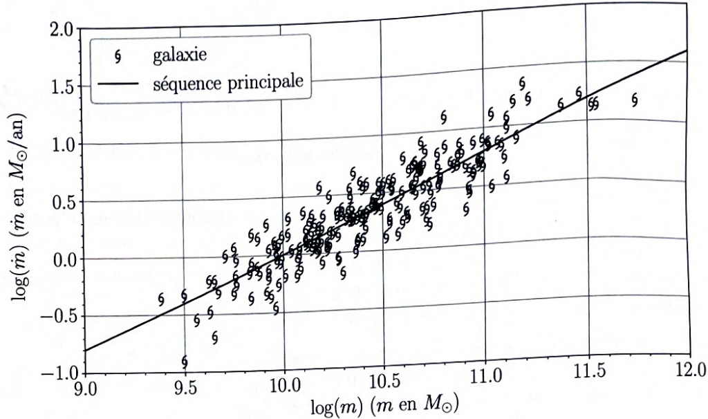
FIGURE 6 – Séquence principale des galaxies
