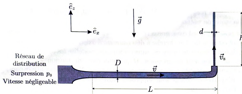
FIGURE 5 – Jet d'eau vertical
