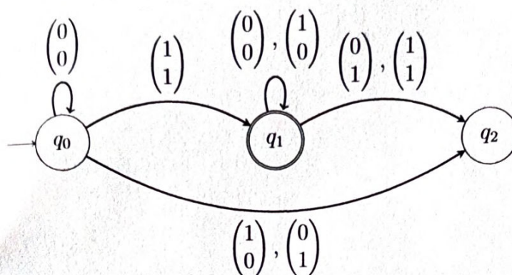
FIGURE 1 – Représentation de l'automate \mathcal{A}_1
