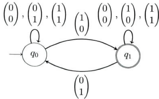
FIGURE 2 – Représentation de l'automate \mathcal{A}_2
